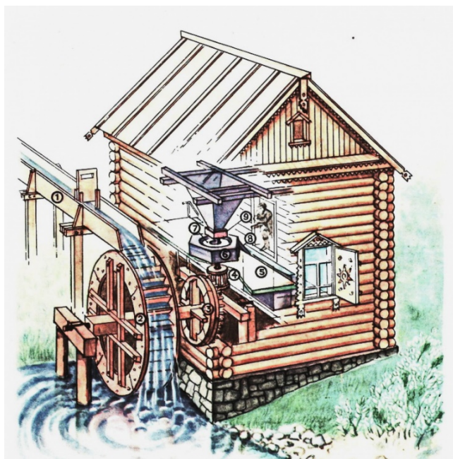
Типовая конструкция водяной мельницы
